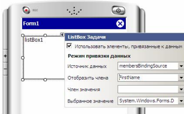
Рис. 3. Привязка ListBox'a к источнику данных.
