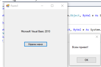
Рис.1.8. Работающая программа.
