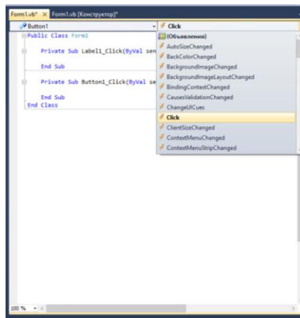
Рис. 1.6. Список объявлений (событий).
