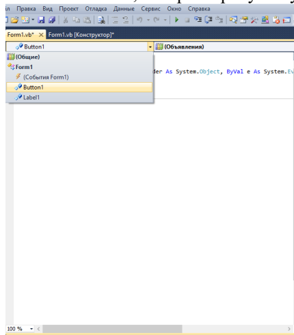
Рис. 1.5. Список объектов.
