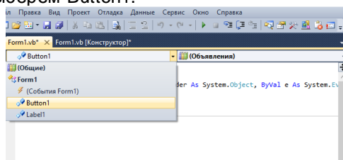
Рис. 1.5. Список объектов.
