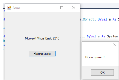
Рис.1.8. Работающая программа.
