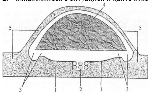
Рис. Геотехсистема по биотермическому обеззараживанию навоза:
